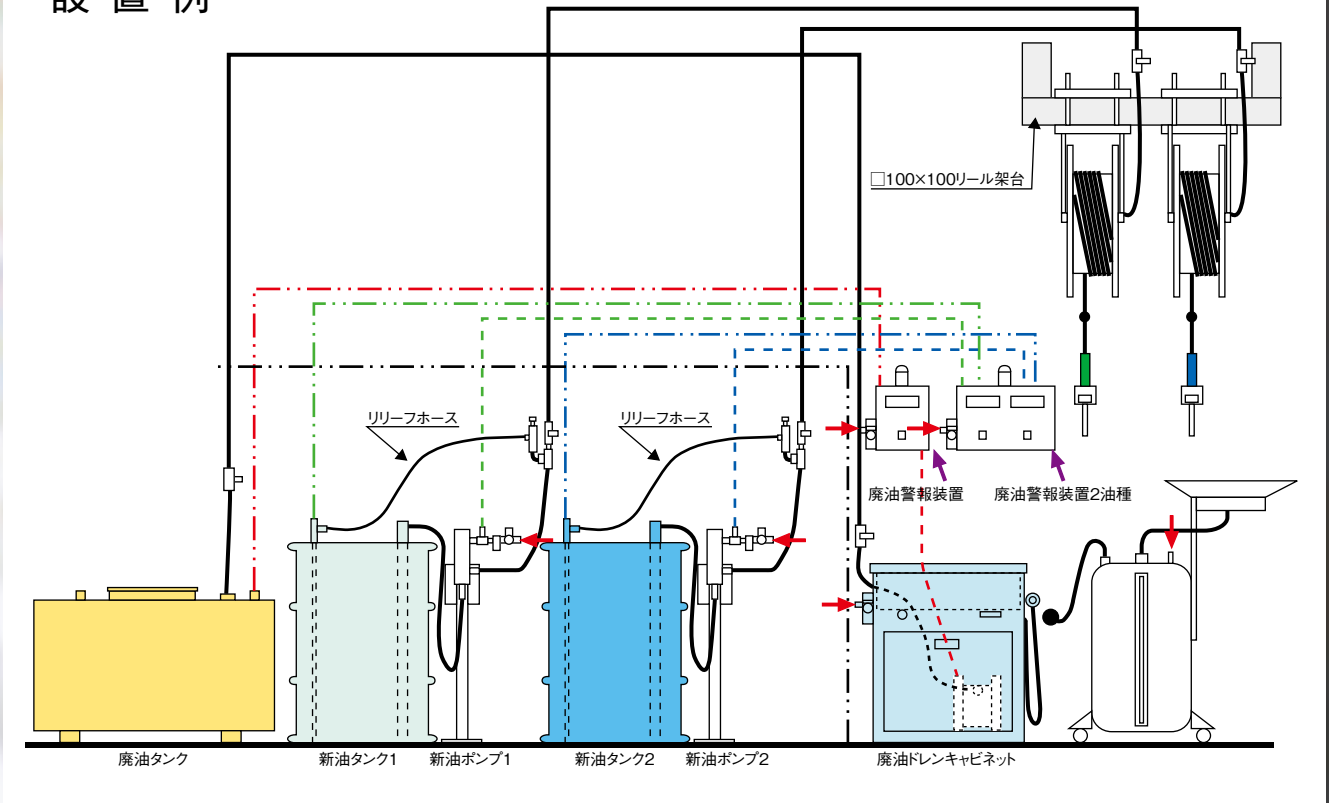
設置例
