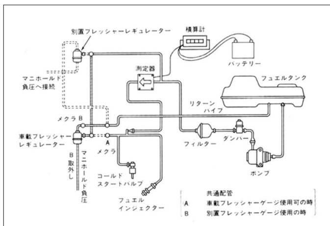
電子制御燃料噴射装置 搭載車両測定時の流量計取付例
