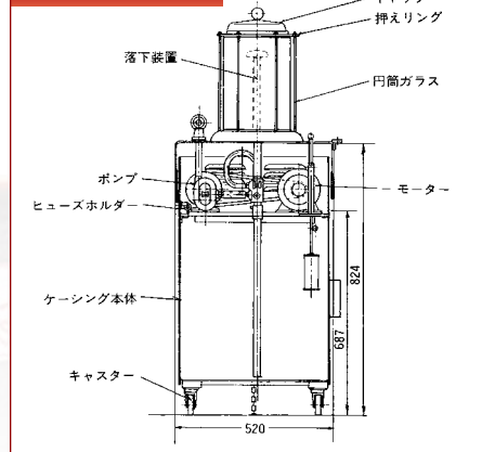
OC-100A 機構図
