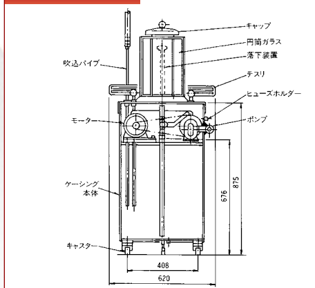
OC-80A 機構図
